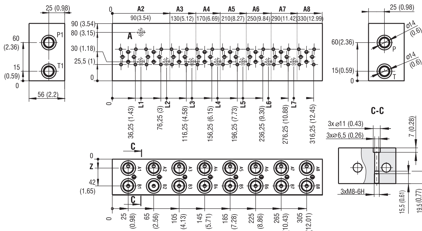
1...8 联的阀块 外形尺寸 单位为毫米 (英寸)
