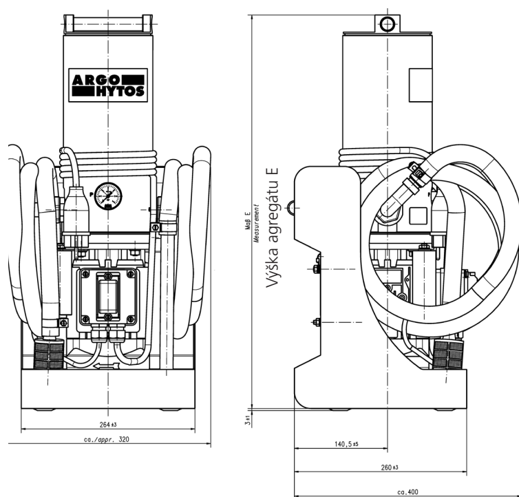
Obr. 11: Rozměry zařízení
