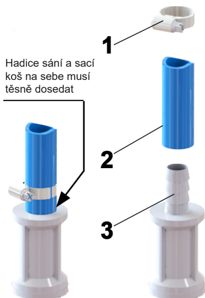
Obr. 4: Výměna sacího koše
