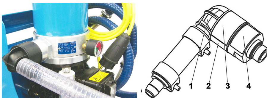
Obr. 10: Volitelné příslušenství "Sada sacích košů"
