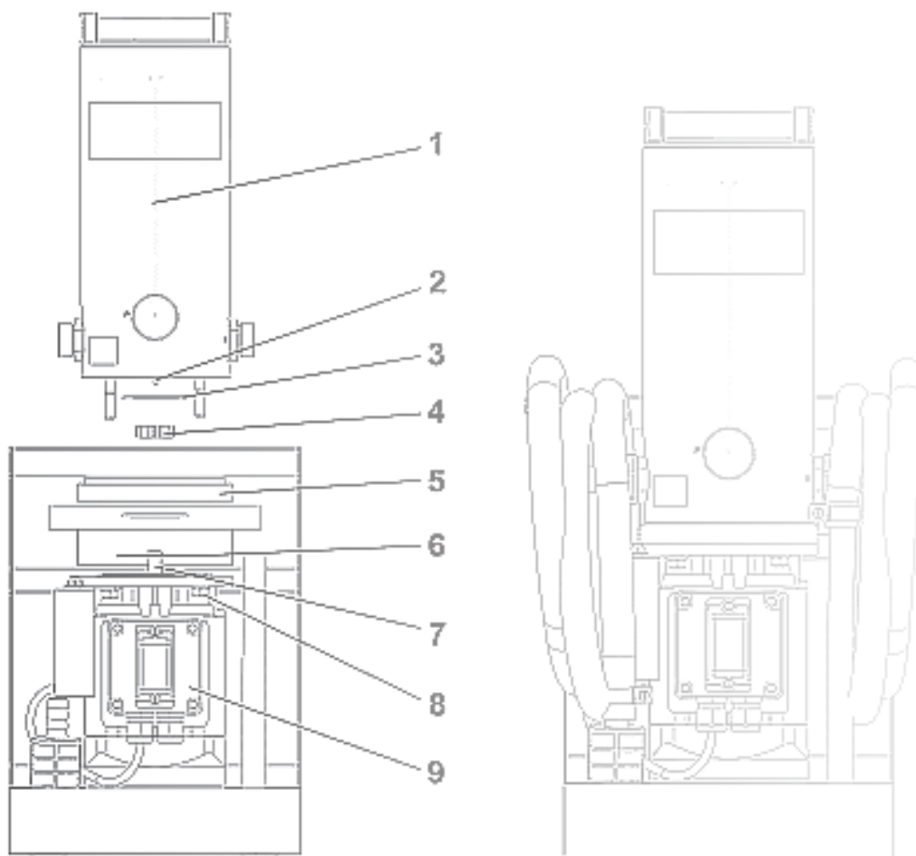
Obr. 9: Výměna motoru a čerpadla
