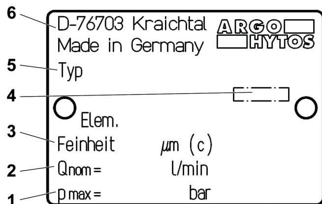
Obr. 2: Štítek
