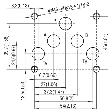
Dn 10 - ISO 4401-05-04-0-05
