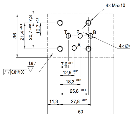
Dn 04 - ISO 4401-AA-02-4-A (DIN 24 340-A4)
