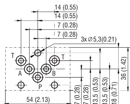
Dn 04 - CETOP-RP 121H
