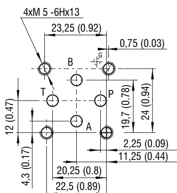
Dn 04 - ISO 4401-02-01-0-05
