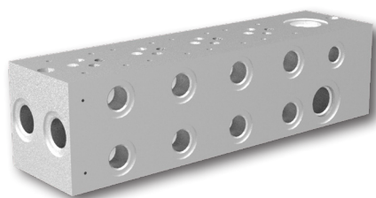
ISO 4401-03-02-0-05
