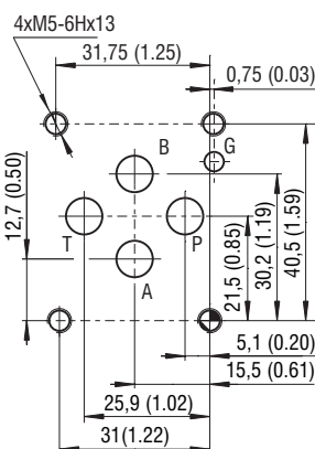
ISO 4401-03-02-0-05
