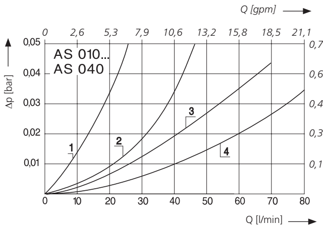
D1 Druckverlust in Abhängigkeit vom Volumenstrom bei v = 35 \text{ mm}^2/\text{s} / 162 \text{ SUS}
