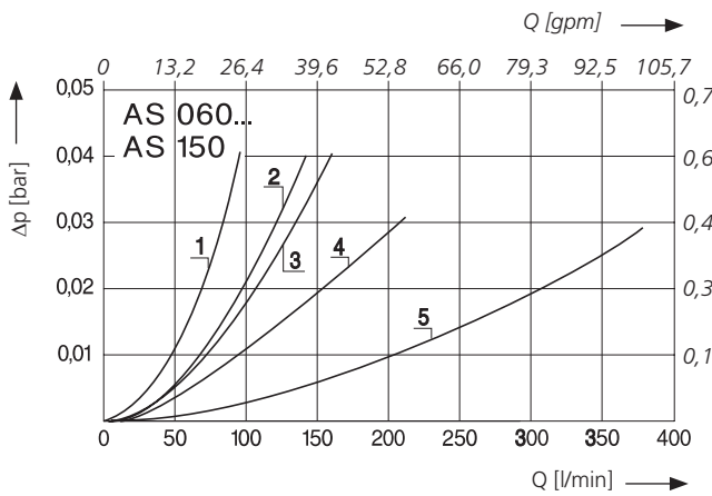
D2 Druckverlust in Abhängigkeit vom Volumenstrom bei v = 35 \text{ mm}^2/\text{s} / 162 \text{ SUS}
