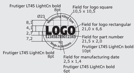
Label Ø26
