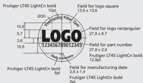
Label Ø33
